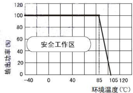
温度曲线图
